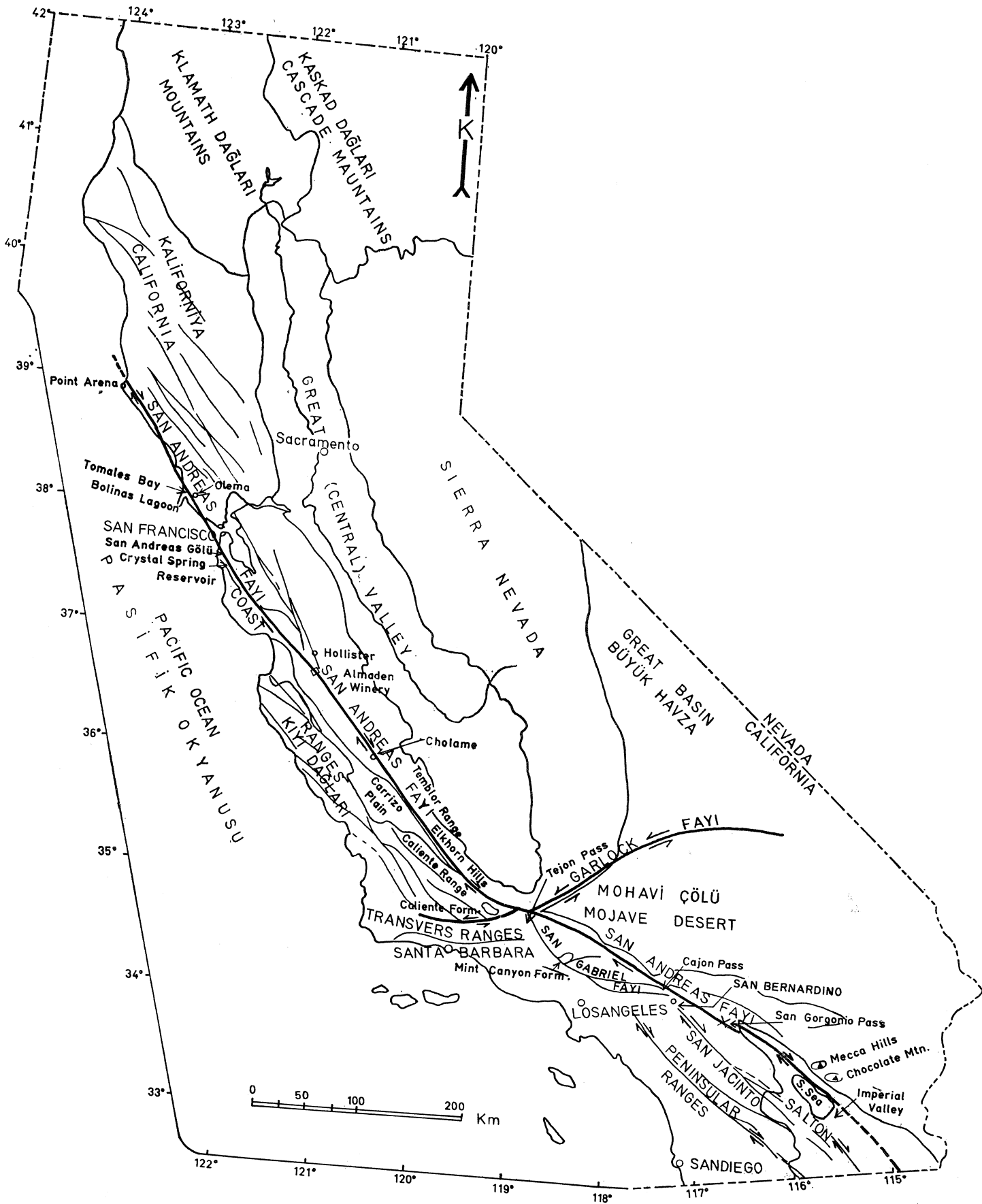
Şekil 1: Kaliforniya'da San Andreas fay zonu. Figure 1: San Andreas fault zone in California.
